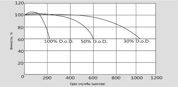
Срок службы в зависимости от глубины разряда
