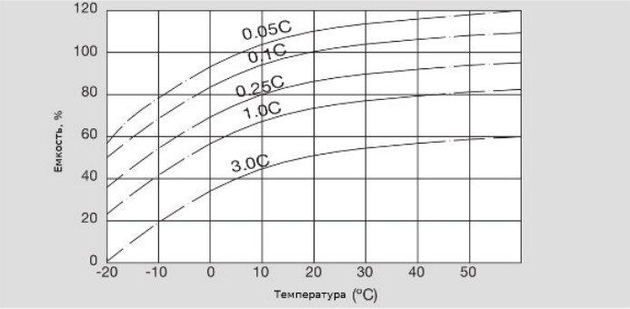
Доступная емкость в зависимости от температуры
